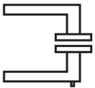
Links Innendrücker mit Schließknopf links zeigend • Für DIN links Türen nach innen öffnend • Für DIN rechts Türen nach außen öffnend
