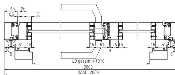
Horizontalschnitt 2-flügelige Stahl-Lofttür
