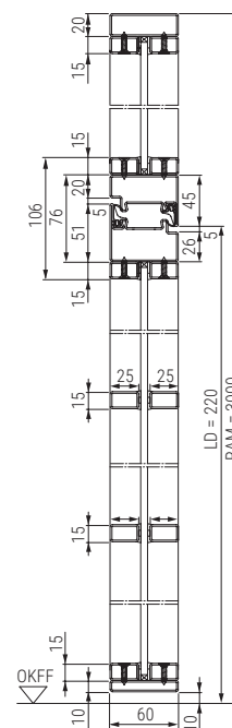
Vertikalschnitt 2-flügelige Stahl-Lofttür mit Oberlicht
