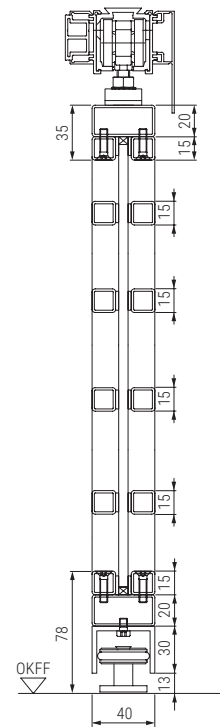
Vertikalschnitt 1-flüglige Stahl-Lofttür
