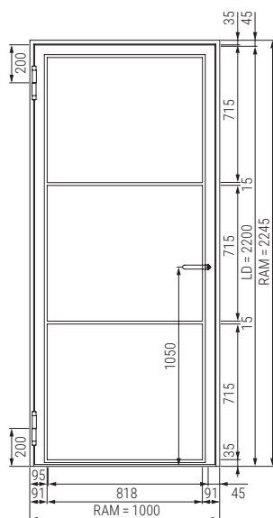
1-flügelige Stahl-Lofttür
