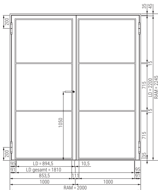
2-flügelige Stahl-Lofttür
