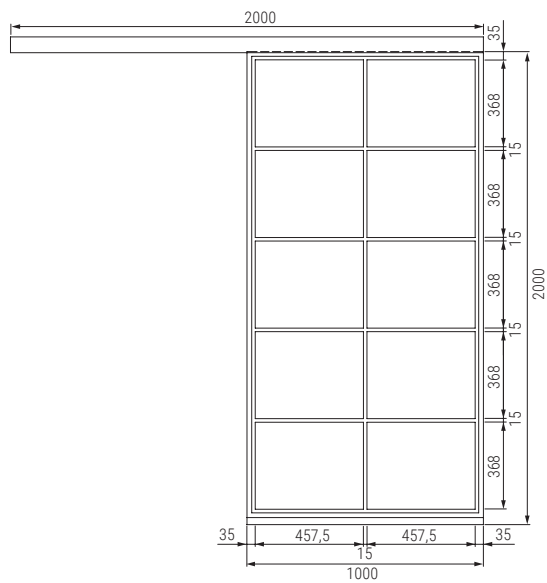
1-flüglige Stahl-Lofttür
