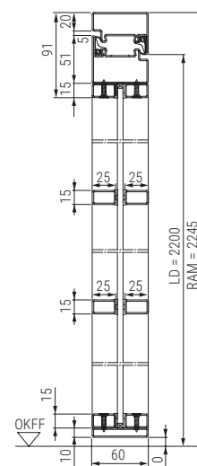
Vertikalschnitt 1-flügelige Stahl-Lofttür
